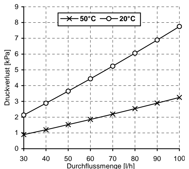
Druckverlustkurven
